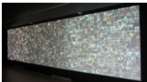
BigData 16.jpg
