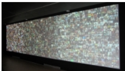
BigData 16.jpg
