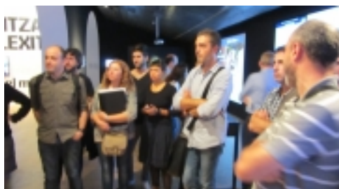
BigData 6.jpg
